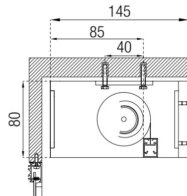
Attacco a soffitto Ceiling mounting
