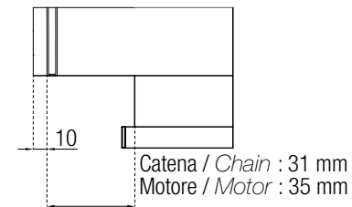
Tolleranza laterale del tessuto Fabric lateral tolerance
