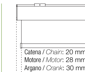
Tolleranza laterale del tessuto Fabric lateral tolerance
