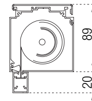
Fondale 15x20 15x20 bottom rail
