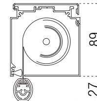
Fondale 19x23 19x23 bottom rail
