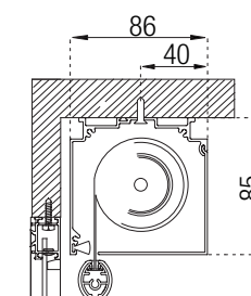
Attacco a soffitto/parete diretto Direct ceiling/wall mounting
