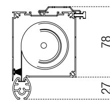
Fondale 19x23 19x23 bottom rail
