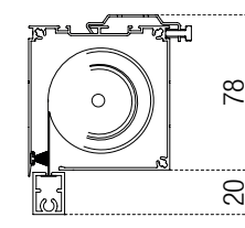
Fondale 15x20 15x20 bottom rail
