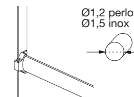
Filo in perlon o inox (opzionali per fondale 19x23) Perlon or stainless steel wire (optionals for 19x23 bottom rail)
