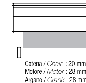
Tolleranza laterale del tessuto Fabric lateral tolerance
